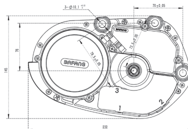
Mid-aandrijf motor
