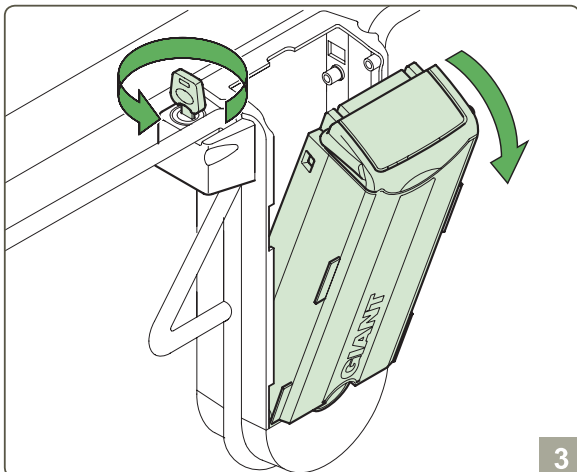
3 Ontgrendel de houder van het EnergyPak en duw het EnergyPak naar buiten.
