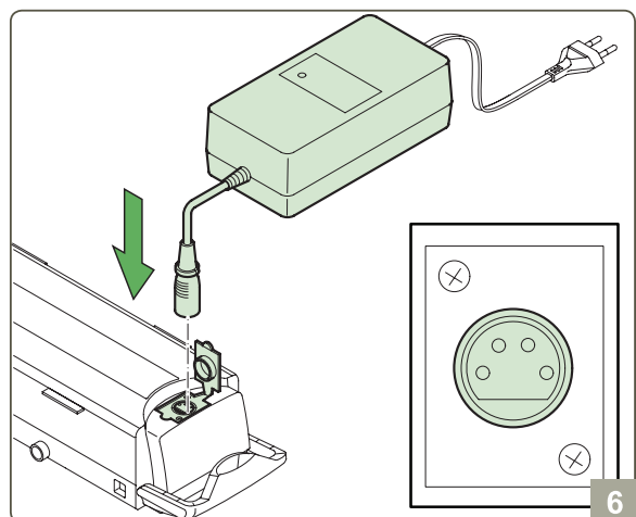
6 Sluit de lader aan op het EnergyPak.
